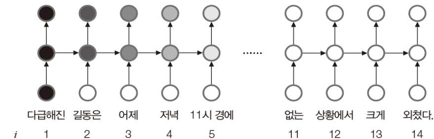
(a) 선별 기억 능력이 없는 순환 신경망
